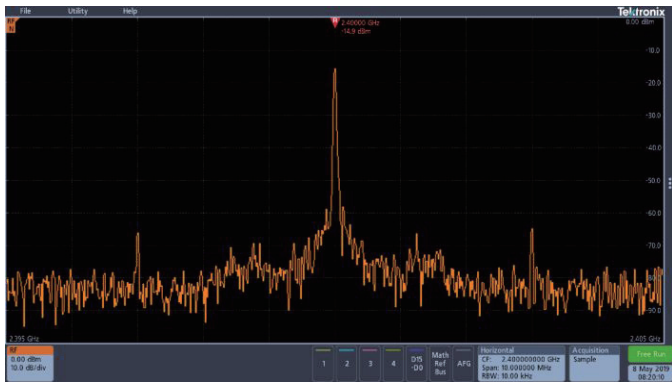
3 系列 MDO 频域显示。
